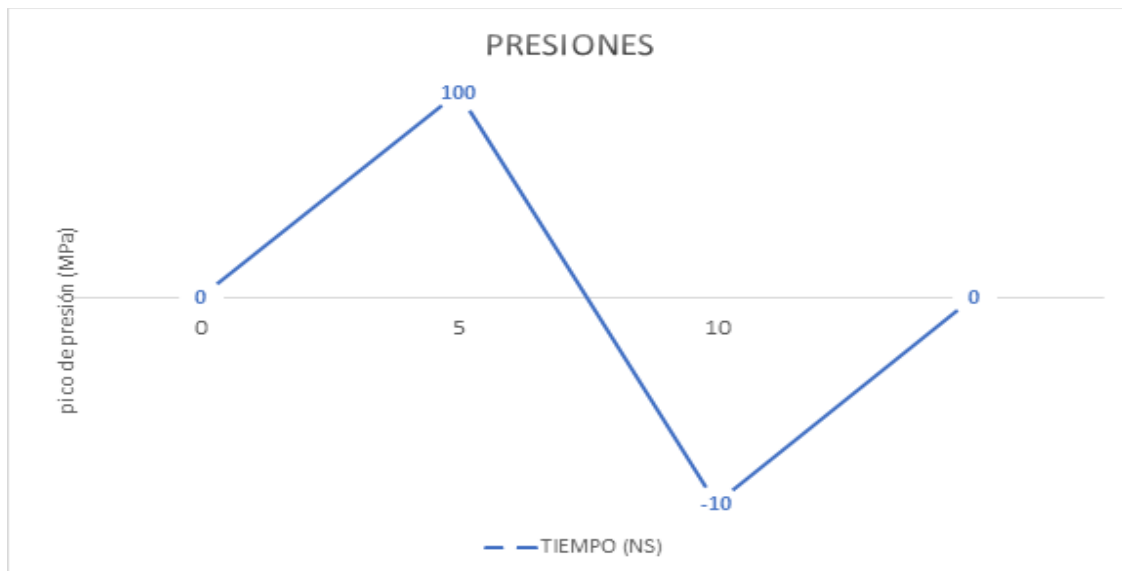
Figura 18. Gráfica de los cambios de presiones en la onda de choque. Elaboración propia.
